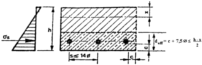
Flessione zone di bordo lastra
