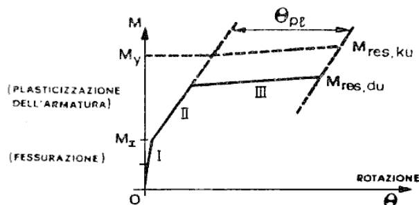
Fig. 1 - Diagramma momento-rotazione: idealizzazione tri-lineare
