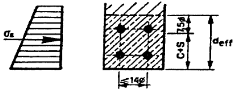
Flessione tratto inferiore anima di trave
