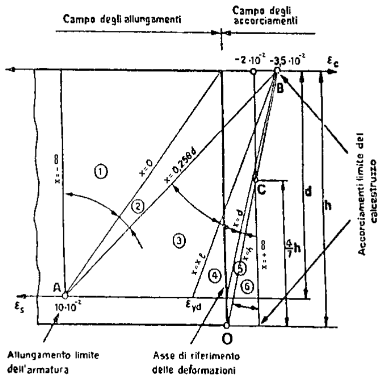
Fig. 2 - Diagramma di deformazione allo stato limite ultimo
