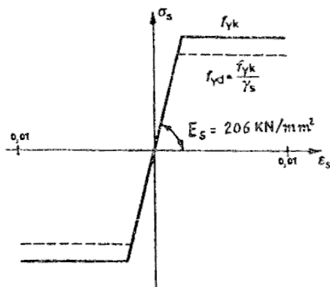
a) acciaio ordinario
