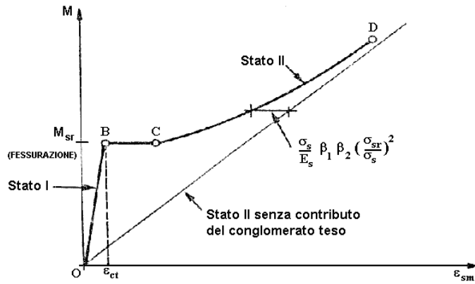
Fig. 6 - Diagramma M - \varepsilon_{sm}
