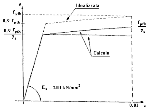
b) acciaio da precompressione
