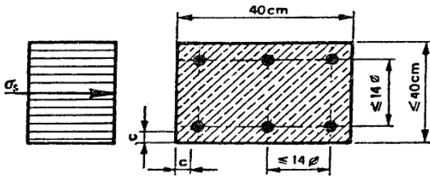
Trazione uniforme travi, solette
