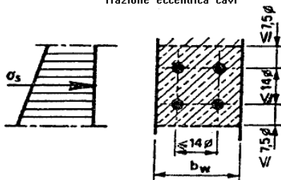
Trazione eccentrica cavi
